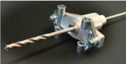
Adaptador para taladrar puertas de madera y poder pasar cables eléctricos ya instalado en el ensamblaje.
